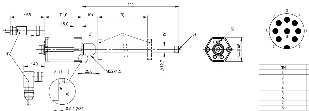
BTL7-S510x-Mxxxx-CD-S32
