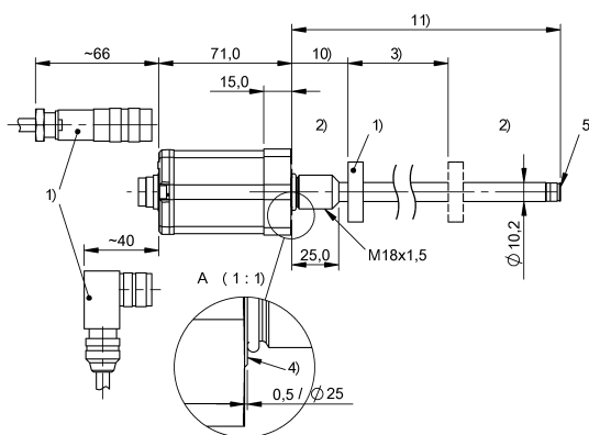
BTL7-P511-Mxxx-B-NEX-S32
