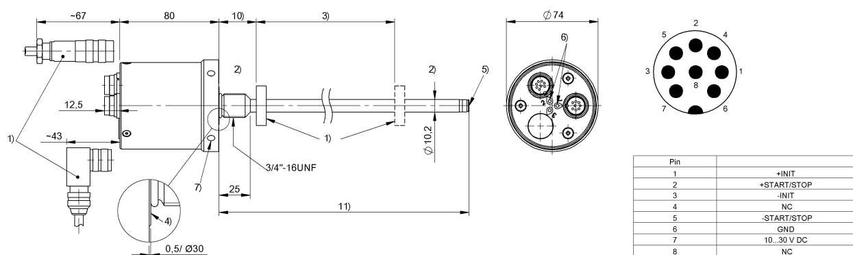
BTL7-P511-Mxxx-TZ2-S32
