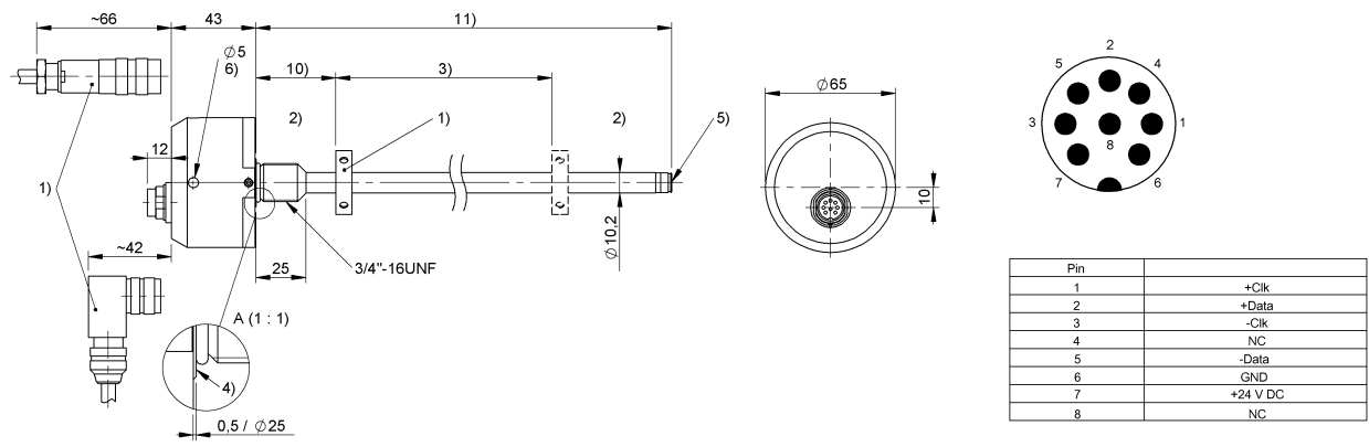
BTL5-Sxxxx-Mxxxx-W-S32
